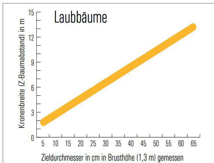
Grafik 1: Zusammenhang Zieldurchmesser mit der Kronenbreite.
