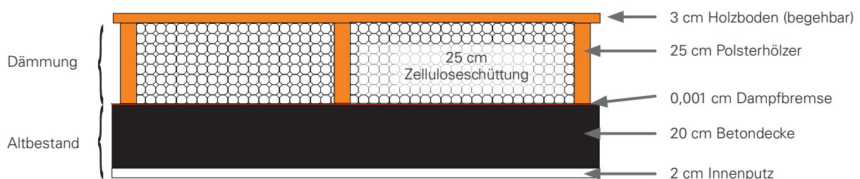
Beispiel einer Dämmung einer Betondecke eins Wohnhauses aus den 70er Jahren
